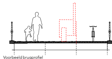
Voorbeeld brugprofiel
