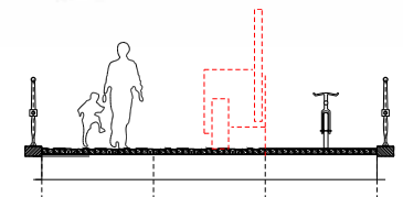
Voorbeeld brugprofiel
