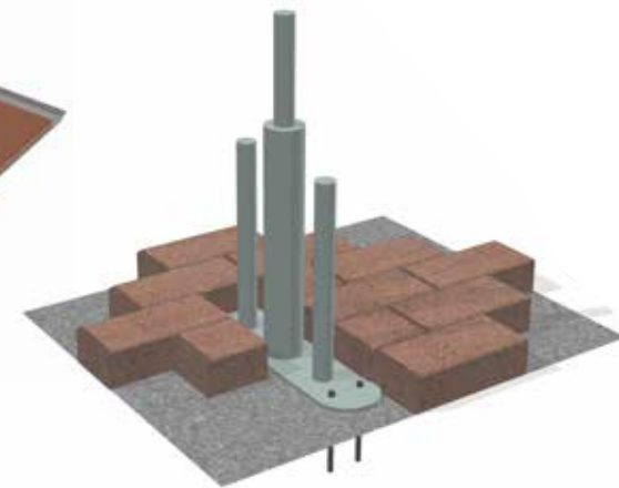
Straatstenen StoneCycling variatie mogelijk in kleur, textuur, hoogte en afkanting van de stenen
